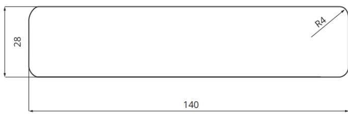
MODŘÍN slezský 28 x 140 mm – detail profilu
